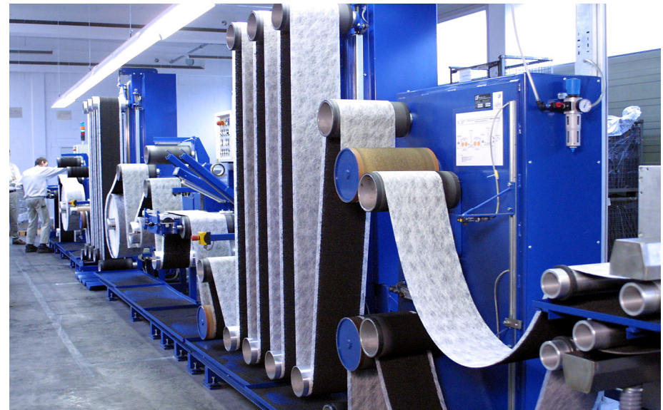
Bandabwicklung FES-Linie
